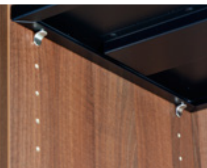
↗ Kovová police s vyztužením – pro skříně šířky 120 cm
